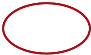
下桶密封圈 Sealing ring 型号 Mode: WG.MF.003.061 尺寸 Size: 内径Φ130×Φ5.3mm
