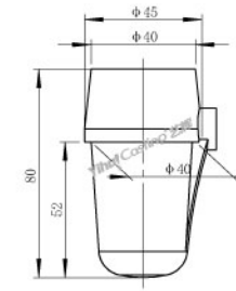
石英齿科坩埚 型号: C.CK.040079 重量: 69g
