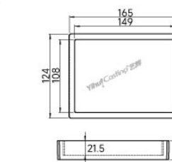
平脚石英焊板 型号: C.CS.00004 重量: 402g
