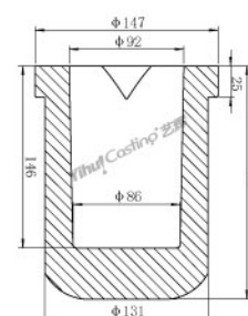
8公斤石英熔金杯 型号: C.CM.B8000 重量: 3000g
