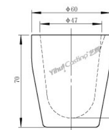
C500石英熔金杯 型号: C.CM.C0500 重量: 136g
