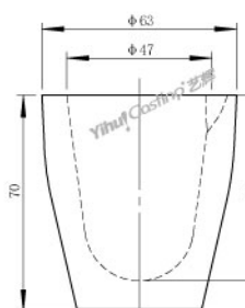
C350石英熔金杯 型号: C.CM.C0350 重量: 144g
