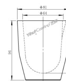
C1000石英熔金杯 型号: C.CM.C1000 重量: 320g
