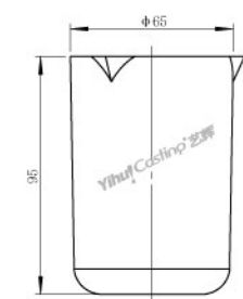
1公斤三嘴石英熔金杯 型号: C.CM.E1000 重量: 245g
