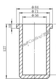
2.5公斤石英外套-F 型号: C.CC.2500F 重量: 292g 2.5kg ceramic shielded-F Model: C.CC.2500F Weight: 292g 包装 Package: 420x315x348mm (40pcs/Carton)
