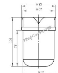
1.5公斤三嘴石英熔金杯 型号: C.CM.A1500 重量: 270g
