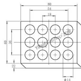
石英配件 型号: C.CA.00011 重量: 177g Ceramic parts Model: C.CA.00011 Weight: 177g
