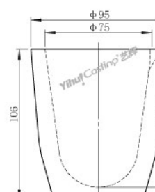
C2000石英熔金杯 型号: C.CM.C2000 重量: 447g
