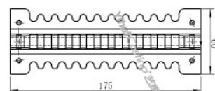
石英发热芯 型号: C.CA.175060 重量: 326g Ceramic heater Model: C.CA.175060 Weight: 326g 包装 Package: 420x315x348mm (52pcs/Carton)
