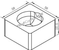
70#石英熔炼方坩埚 型号: C.CM.00070 重量: 98g
