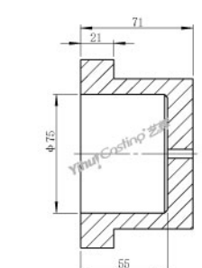
4公斤石英底座 型号: C.CD.04000 重量: 787g 4kg ceramic base Model: C.CD.04000 Weight: 787g 包装 Package: 450x300x240mm (22pcs/Carton)
