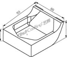
73#石英熔炼方坩埚 型号: C.CM.00073 重量: 222g
