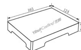
4脚石英焊板 型号: C.CS.00001 重量: 357g
