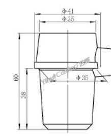
石英齿科坩埚 型号: C.CK.035061-B 重量: 54g
