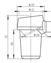
石英齿科坩埚 型号: C.CK.038075-A 重量: 61g
