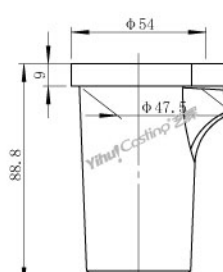
600克石英熔金杯 型号: C.CM.B0600 重量: 139g
