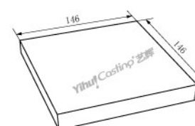
石英盖板 型号: C.CS.00016 重量: 735g
