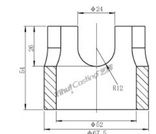
石英配件 型号: C.CA.00012 重量: 111g Ceramic parts Model: C.CA.00012 Weight: 111g
