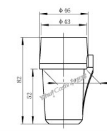
石英齿科坩埚 型号: C.CP.YK-F1 重量: 79g
