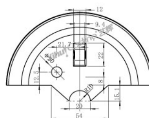
石英前盖 型号: C.CA.00008-B 重量: 148g Ceramic front cover Model: C.CA.00008-B Weight: 148g
