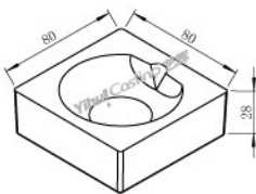
72#石英熔炼方坩埚 型号: C.CM.00072 重量: 237g
