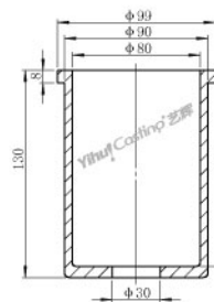
4公斤石英外套 (底孔30mm) 型号: C.CC.4000A-30 重量: 378g 4kg ceramic shielded (Bottom hole 30mm) Model: C.CC.4000A-30 Weight: 378g 包装 Package: 420x315x348mm (24pcs/Carton)
