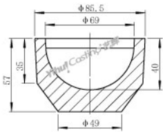
石英熔炼坩埚 型号: C.CM.086056 重量: 287g
