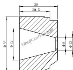
K2-SM1石英铸造坩埚底座 型号: C.CD.K0050 重量: 117g K2-SM1 Ceramic casting crucible base Model: C.CD.K0050 Weight: 117g
