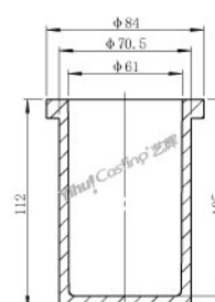
2公斤石英外套 型号: C.CC.2000A 重量: 265g 2kg ceramic shielded Model: C.CC.2000A Weight: 265g 包装 Package: 450x300x240mm (30pcs/Carton)
