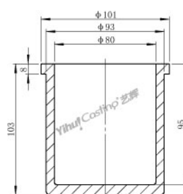
石英熔炼坩埚 型号: C.CC.093103 重量: 395g Ceramic melting crucible Model: C.CC.093103 Weight: 395g
