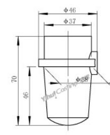
石英齿科坩埚 型号: C.CK.037071-A 重量: 64g
