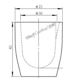
C750石英熔金杯 型号: C.CM.C0750 重量: 255g
