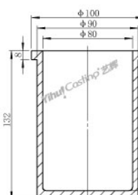
4公斤石英外套-A 型号: C.CC.4000A 重量: 392g 4kg ceramic shielded-A Model: C.CC.4000A Weight: 392g 包装 Package: 420x315x348mm (24pcs/Carton)
