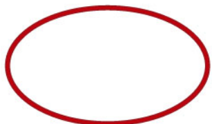
O型密封圈 O-Sealing ring 型号 Mode: WG.MF. 003.189 尺寸 Size: 内径 Inner Diameter Φ206×Φ7mm
