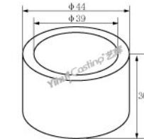
石英熔炼坩埚 型号: C.CM.00005-0SCT 重量: 70g
