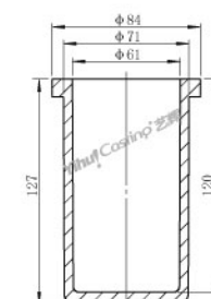
2.5公斤石英外套-A 型号: C.CC.2500A 重量: 292g 2.5kg ceramic shielded-A Model: C.CC.2500A Weight: 292g 包装 Package: 420x315x348mm (40pcs/Carton)
