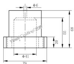
1公斤石英底座 型号: C.CD.01000 重量: 300g 1kg ceramic base Model: C.CD.01000 Weight: 300g 包装 Package: 450x300x240mm (45pcs/Carton)
