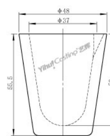
C200石英熔金杯 型号: C.CM.C0200 重量: 64g
