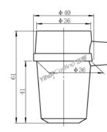
石英齿科坩埚 型号: C.CK.035061-A 重量: 48g
