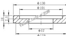
2公斤、3公斤石英法兰 型号: C.CA.02055 重量: 314g 2kg/3kg ceramic flange Model: C.CA.02055 Weight: 314g 包装 Package: 420x315x348mm (90pcs/Carton)
