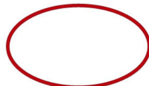
O型密封圈 O-Sealing ring 型号 Mode: WG.MF. 003.189 尺寸 Size: 内径 Inner Diameter \Phi 206 \times \Phi 7\text{mm}
