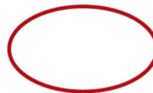
下桶密封圈 Sealing ring 型号 Mode: WG.MF.003.061 尺寸 Size: 内径 \Phi 130 \times \Phi 5.3\text{mm}
